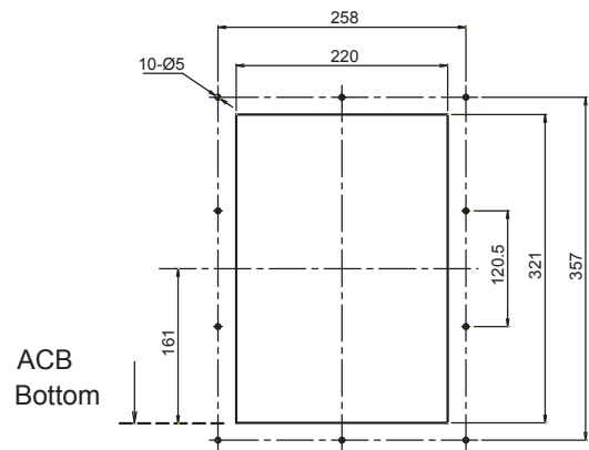
Door Frame Dimensions
